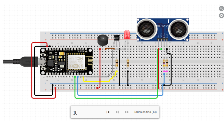
Figura 7 – Fonte: circuito.io.
