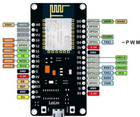
Figura 2 – Placa NodeMCU ESP8266_ pinagem. Fonte: AranaCorp.
