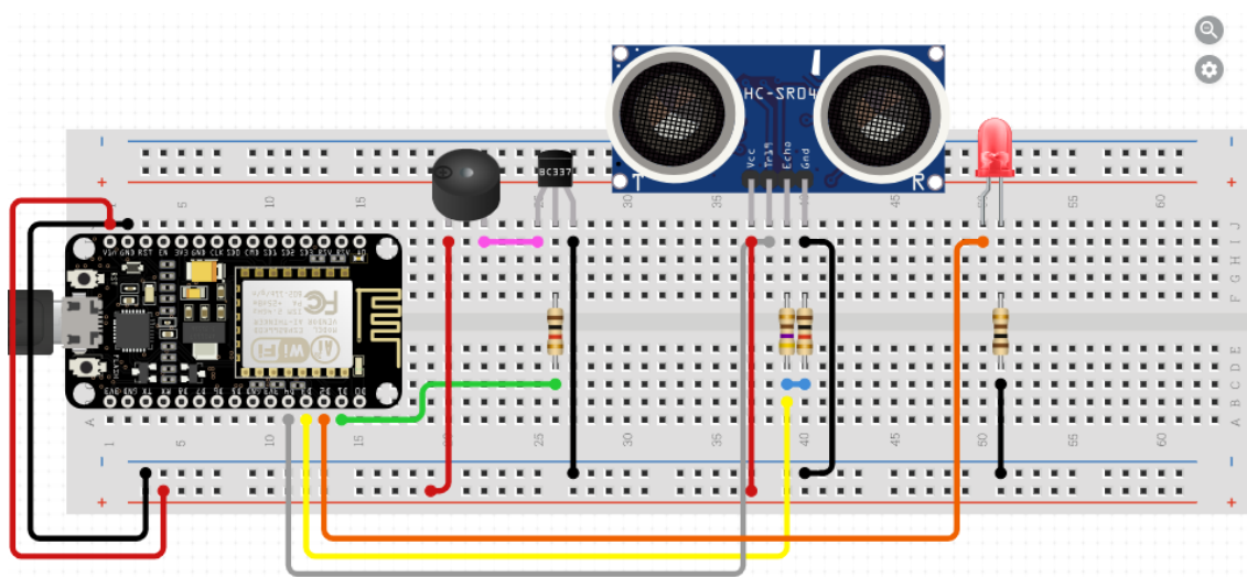
Figura 9 – Diagrama de montagem do protótipo.
