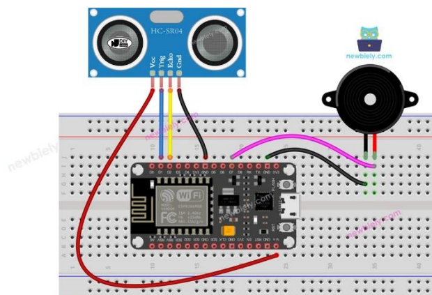
Figura 6 – Buzzer. Fonte: NewBiely.
