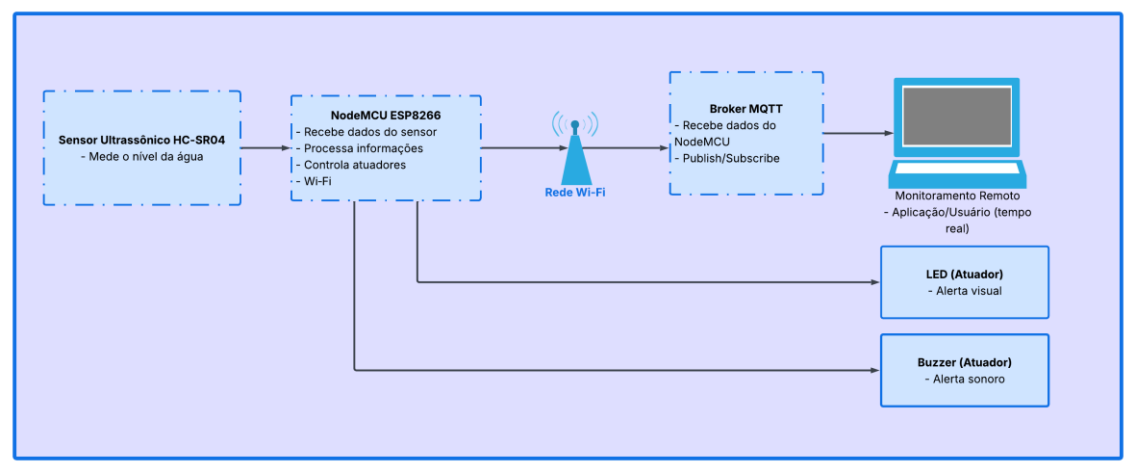
- Figura 13 – Arquitetura MQTT.
