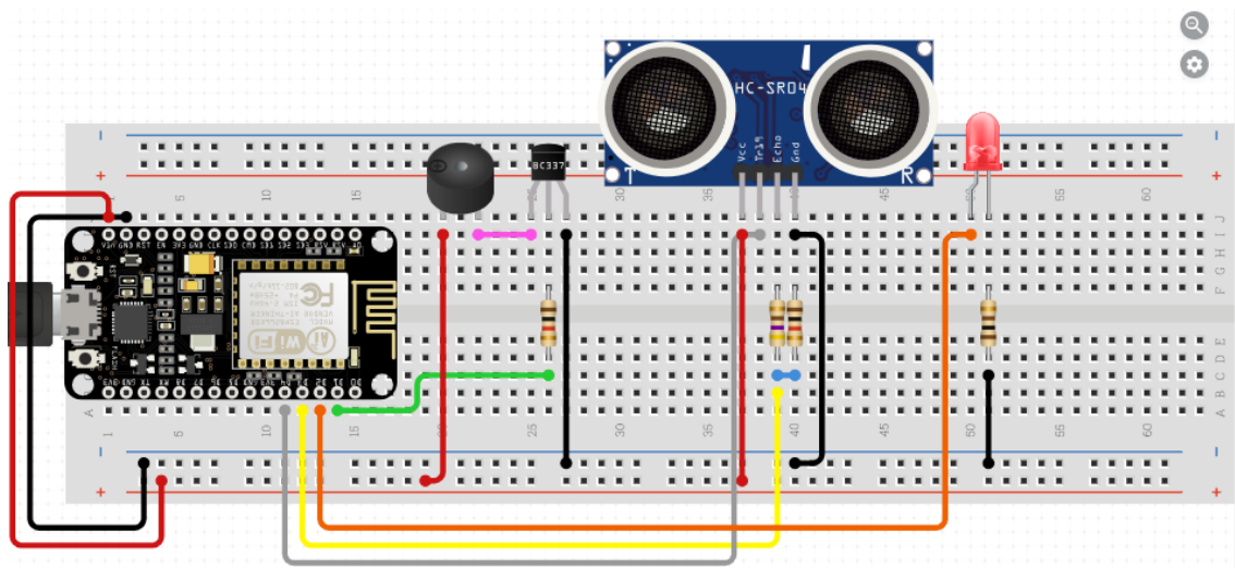
- Figura 11 – Diagrama de montagem do sistema.
