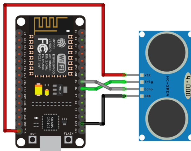
Figura 4 – NodeMCU_HC-SR04. Fonte: RandomNerdTutorials.
