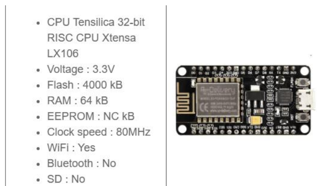
Figura 1 – Placa NodeMCU ESP8266: AranaCorp.
