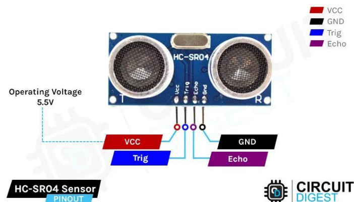
Figura 3 – HC-SR04. Fonte: CircuitDigest.
